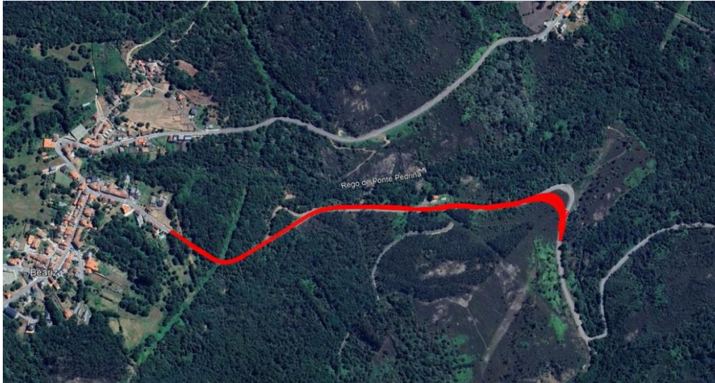
Treito de actuación en Beariz con rectificación da curva do quilómetro 7+350
