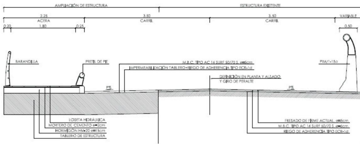
SECCIÓN TIPO EN ESTRUCTURA Escala 1:50
