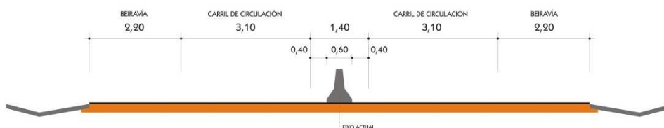
SECCION TRONCO . SECCION PROPOSTA
