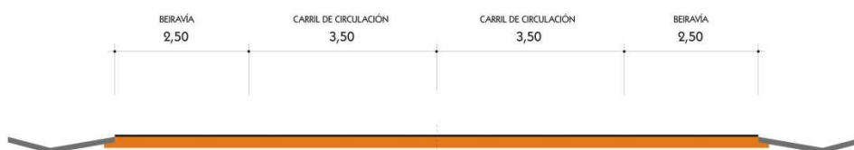
SECCION TRONCO . SECCION PROPOSTA
